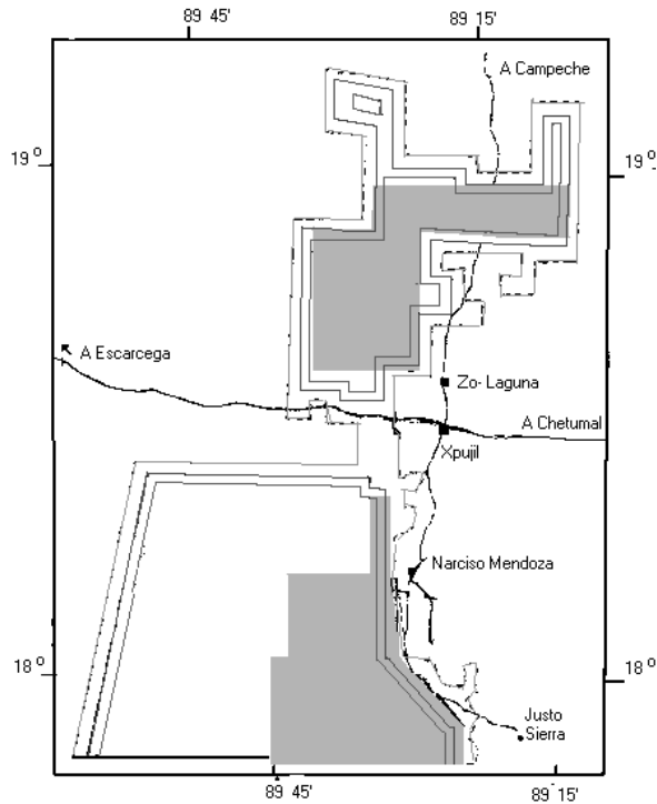
Figura 3. Pérdidas de área estimadas bajo efectos de borde de 3 y 5 km en la Reserva de la Biosfera de Calakmul, Campeche, México.
