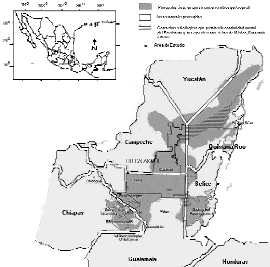
Figura 1. Ubicación del sitio de estudio en la Reserva de la Biosfera de Calakmul, Campeche, México.
